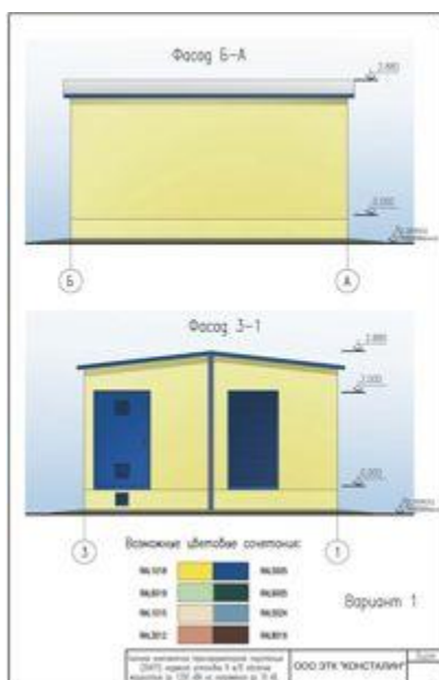
2BKTTP-1000 бетонная подстанция Нажмите на картинку для увеличения
