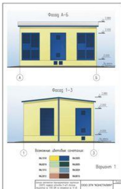
2БКТП-1000 бетонная подстанция Нажмите на картинку для увеличения
